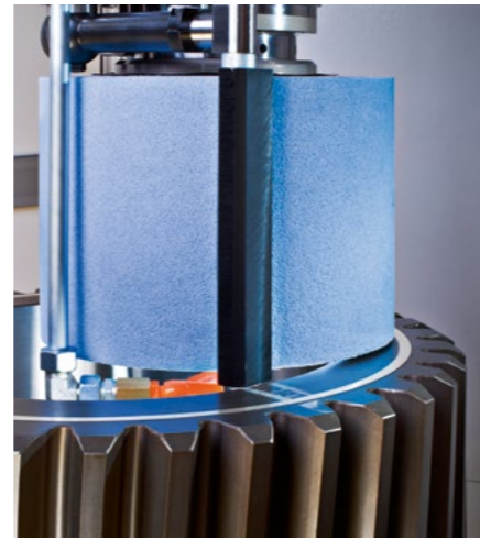
ZP I/E mit schnell wendbarem Schleifarm für die Bearbeitung großmoduliger Innen- und Außenverzahnungen
